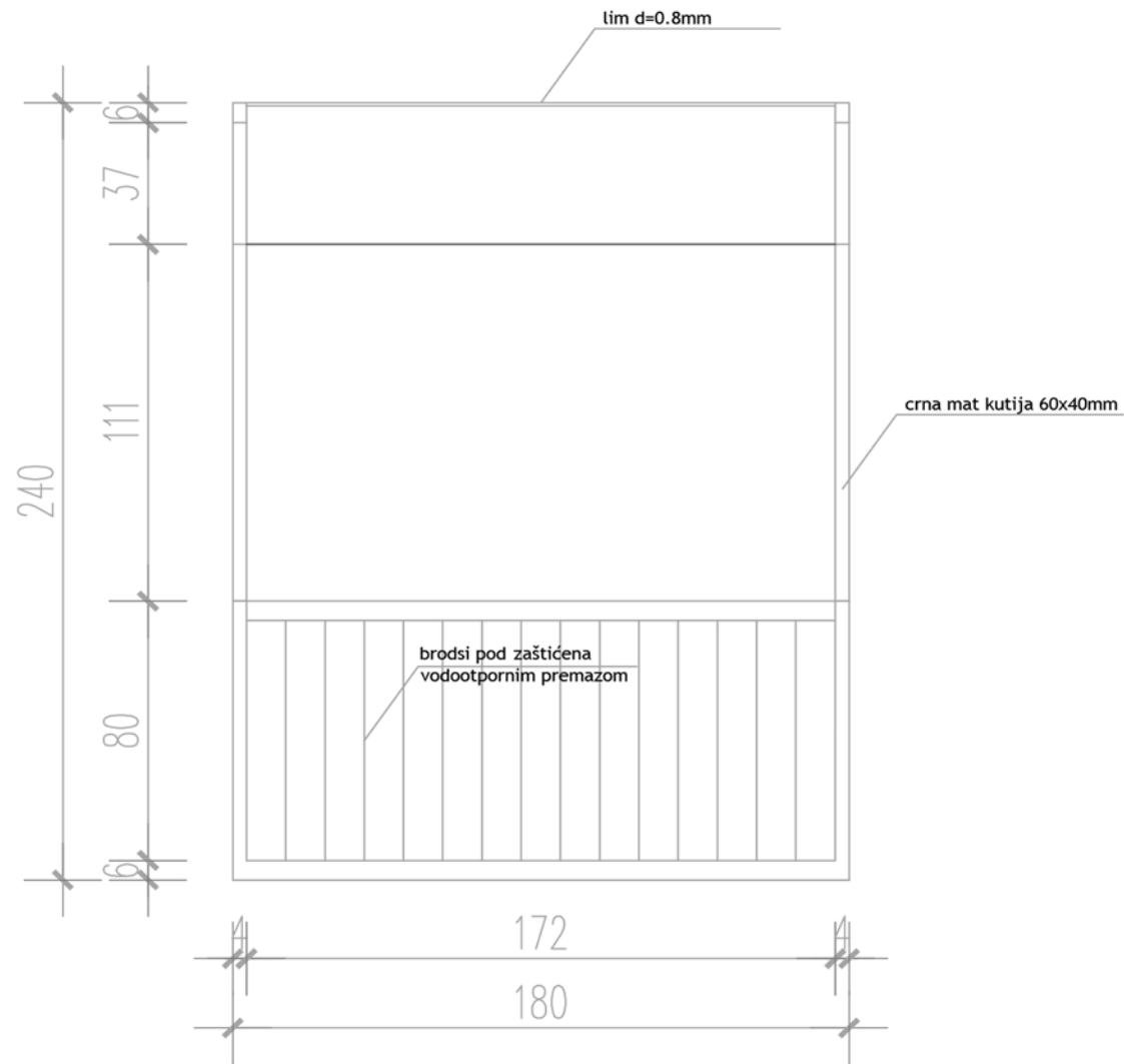
izgled.
