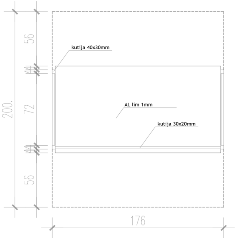
osnova.
