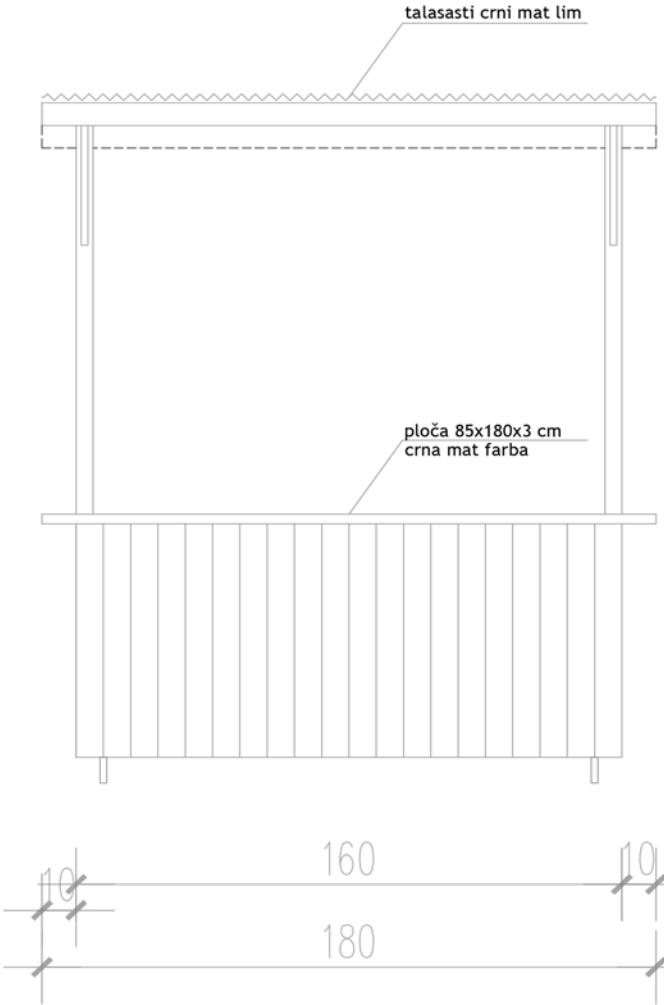
izgled.
