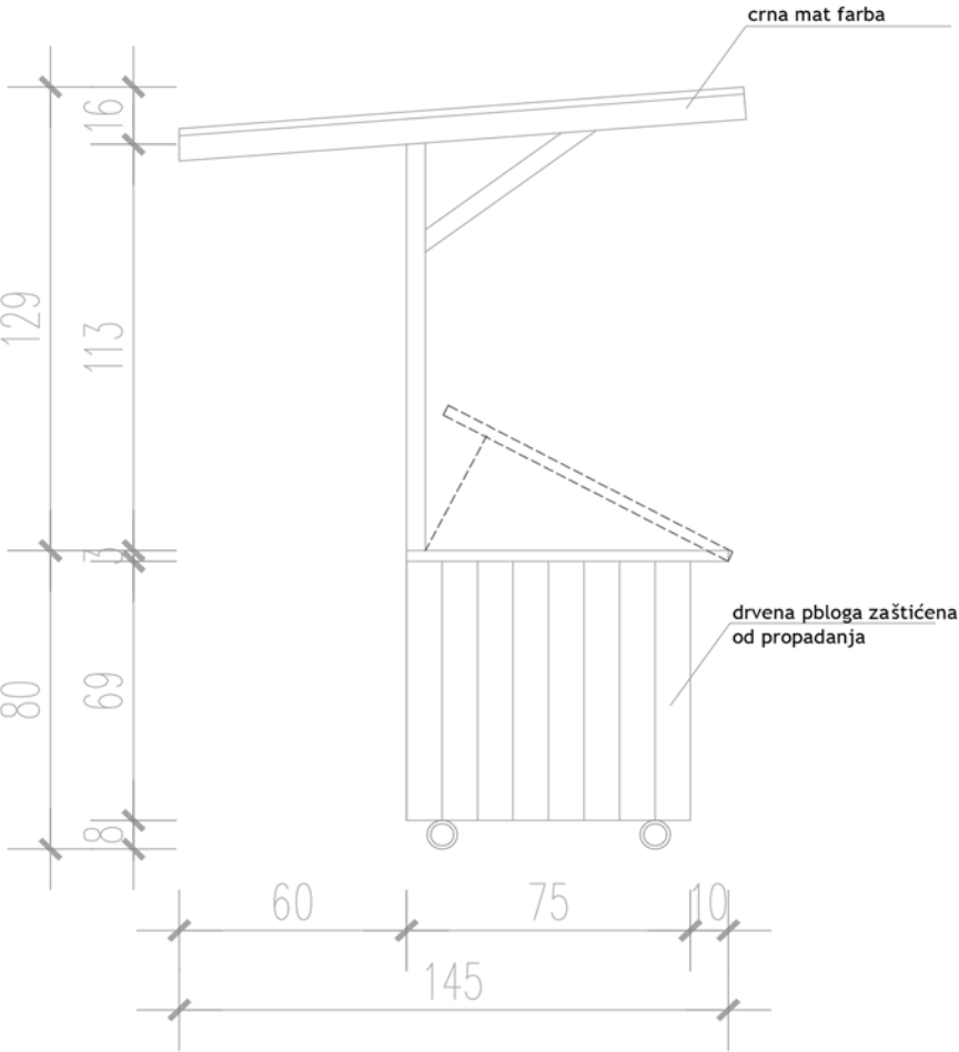
presek a.
