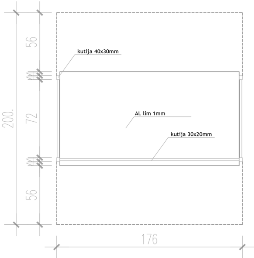
osnova.
